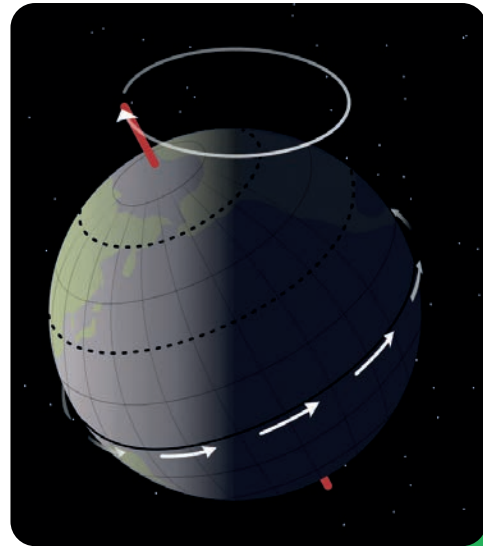
Movimento de rotação da Terra que define as horas do dia.
